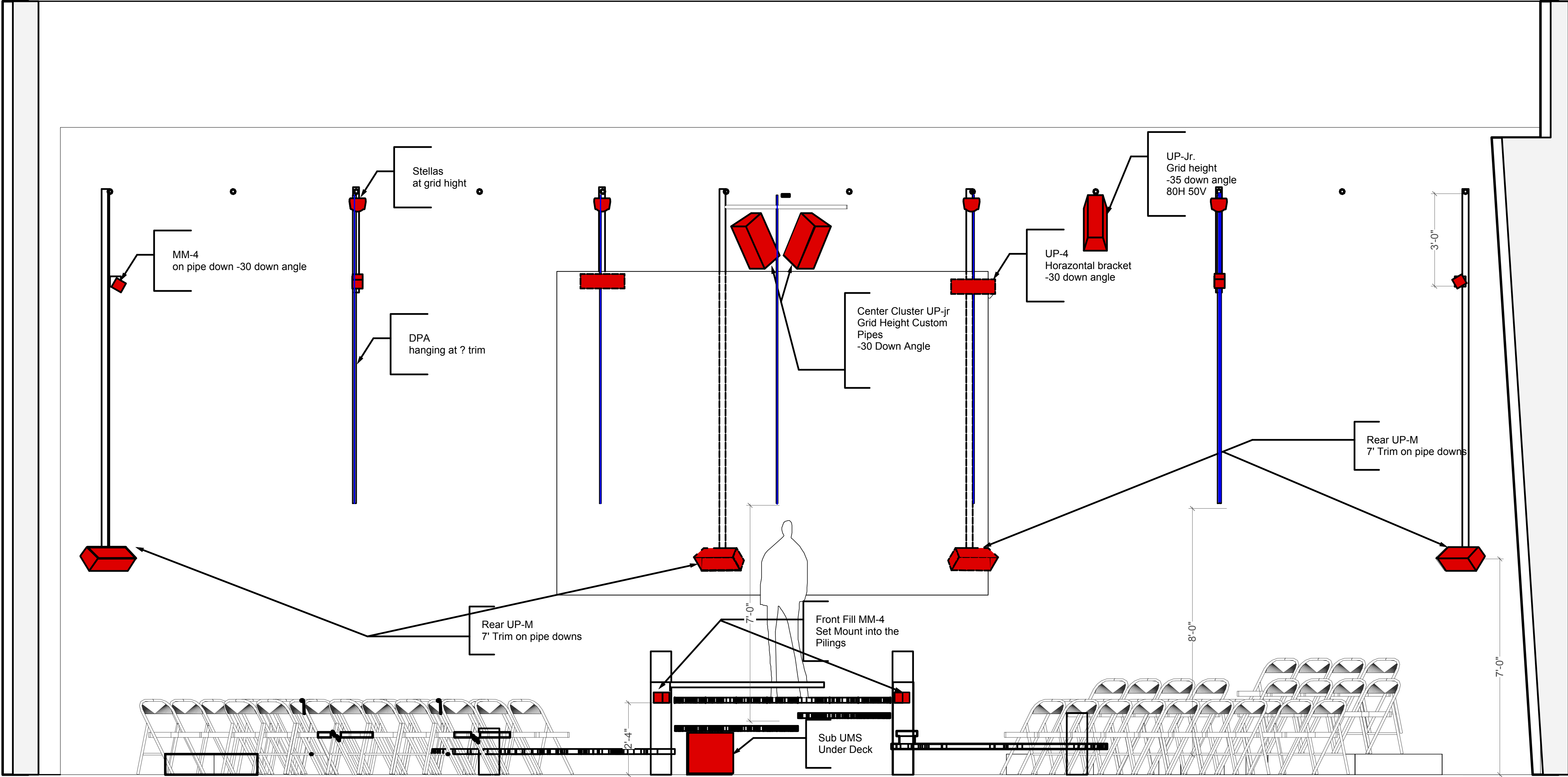
1 SND section Scale: 1/2" = 1'-0"
